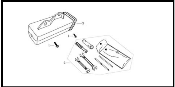
F-32 HERRAMIENTAS
