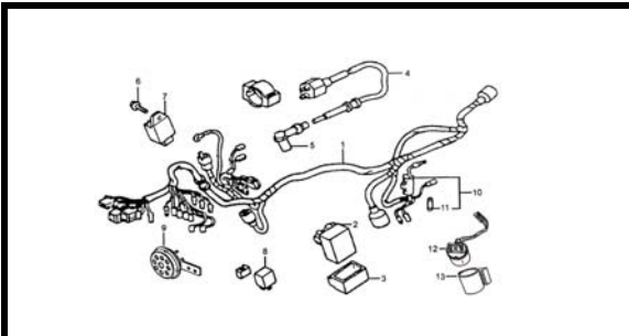
F-28 SISTEMA ELÉCTRICO
