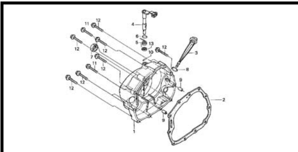
E-7-1 BOMBA LUBRICACIÓN
