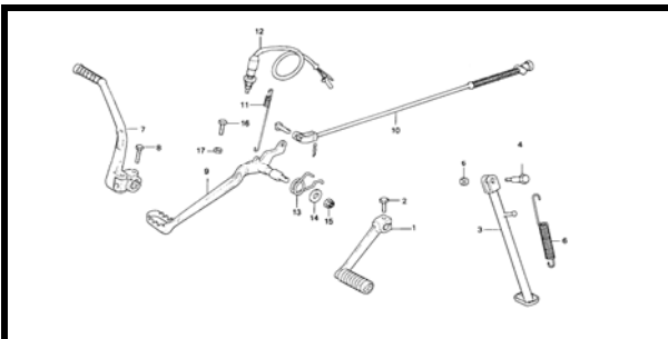
F-20 PEDAL FRENO
