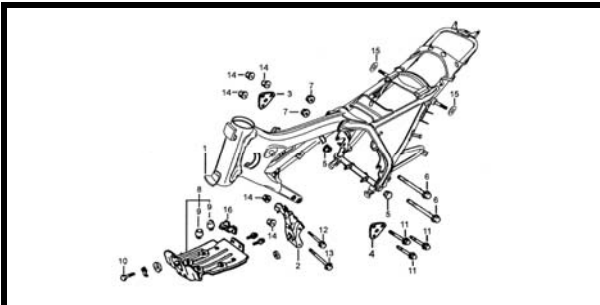
F-29 CHASIS
