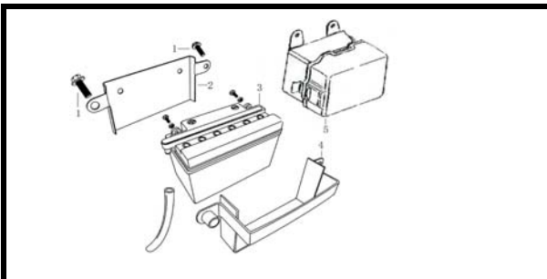
F-29 CHASIS
