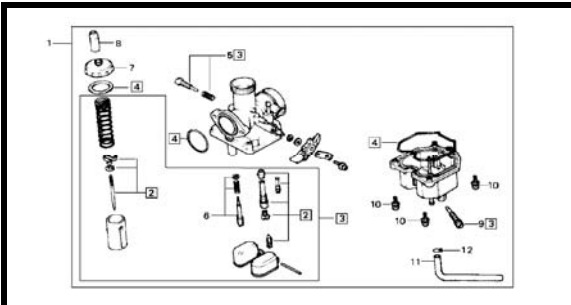
F-1 CARBURADOR
