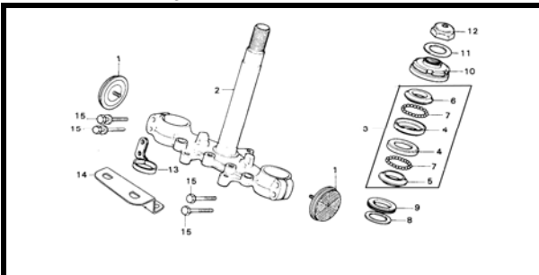
F-8 SUSPENSIÓN DELANTERA
