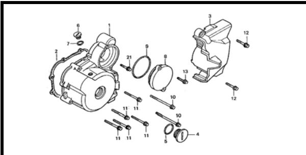
E-8 CUBIERTA IZQUIERDA
