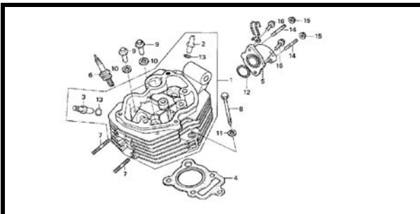
E-4 CILINDRO
