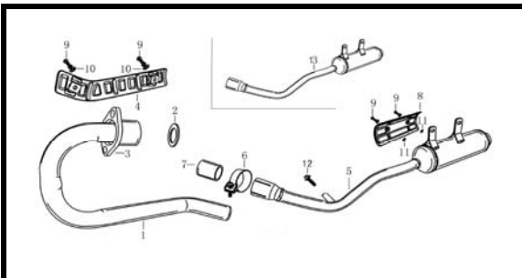
F-19 MOFLE
