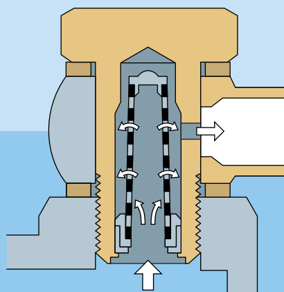
Estrangulador de retorno
