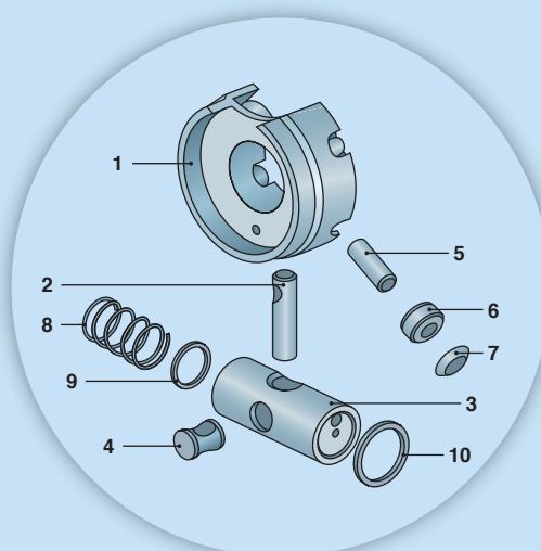
Componentes do conjunto
