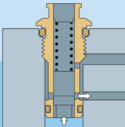
Válvula reguladora de pressão
