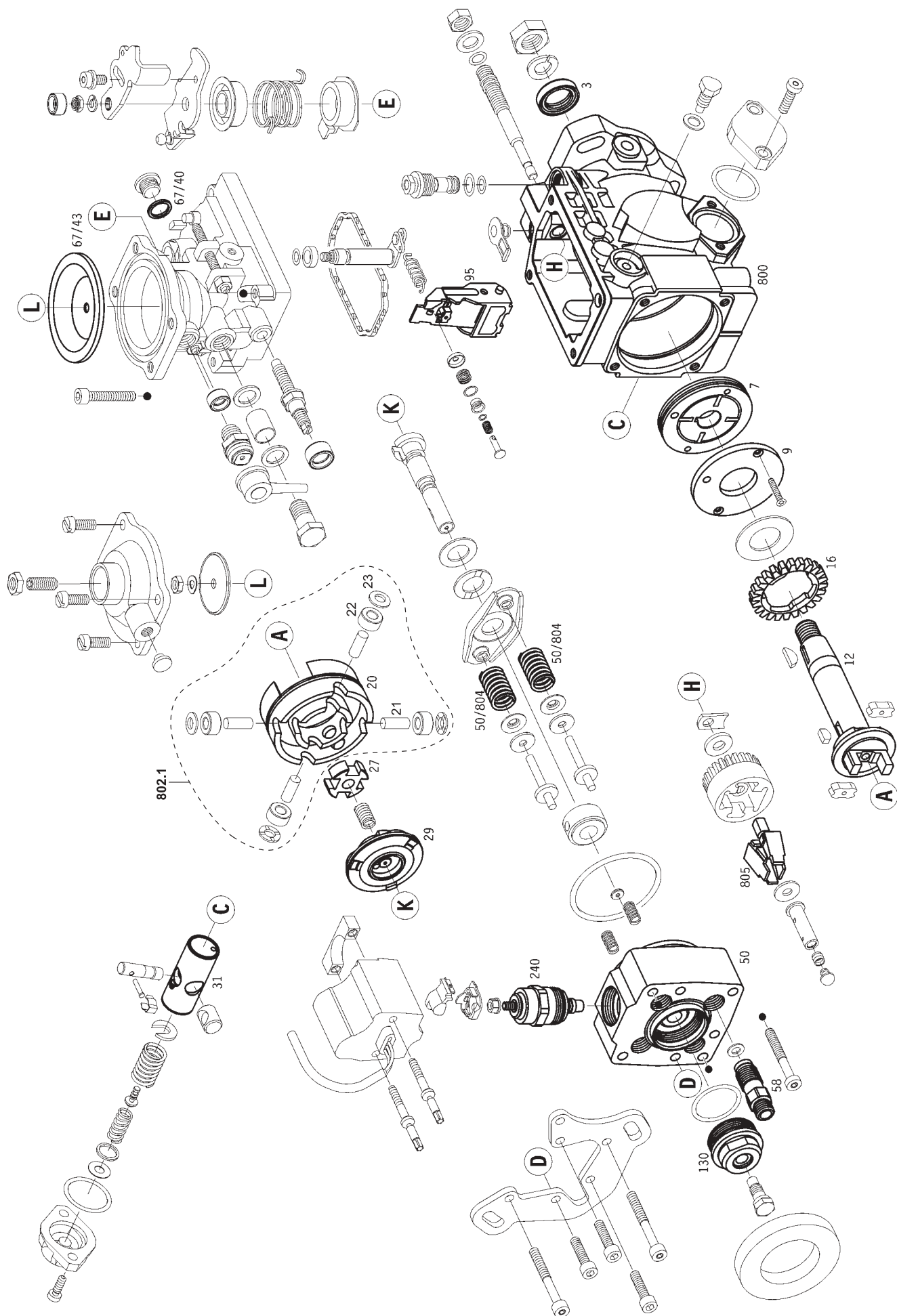
Bombas distribuidoras VE: 0 460 424 222 Bombas de inyección rotativa VE: 0 460 424 223
