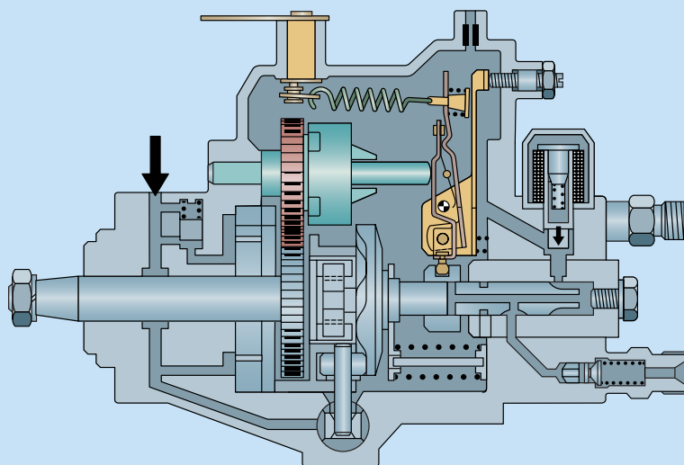
Bomba distribuidora com conjunto regulador, que consiste de regulador de força centrífuga e conjunto de alavancas
