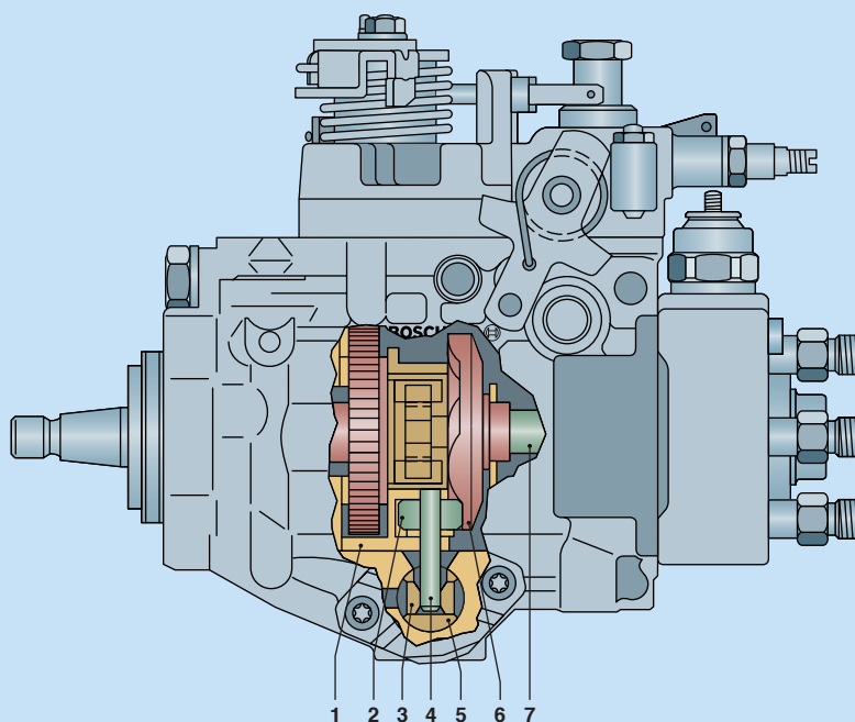
Bomba distribuidora com avanço de injeção
