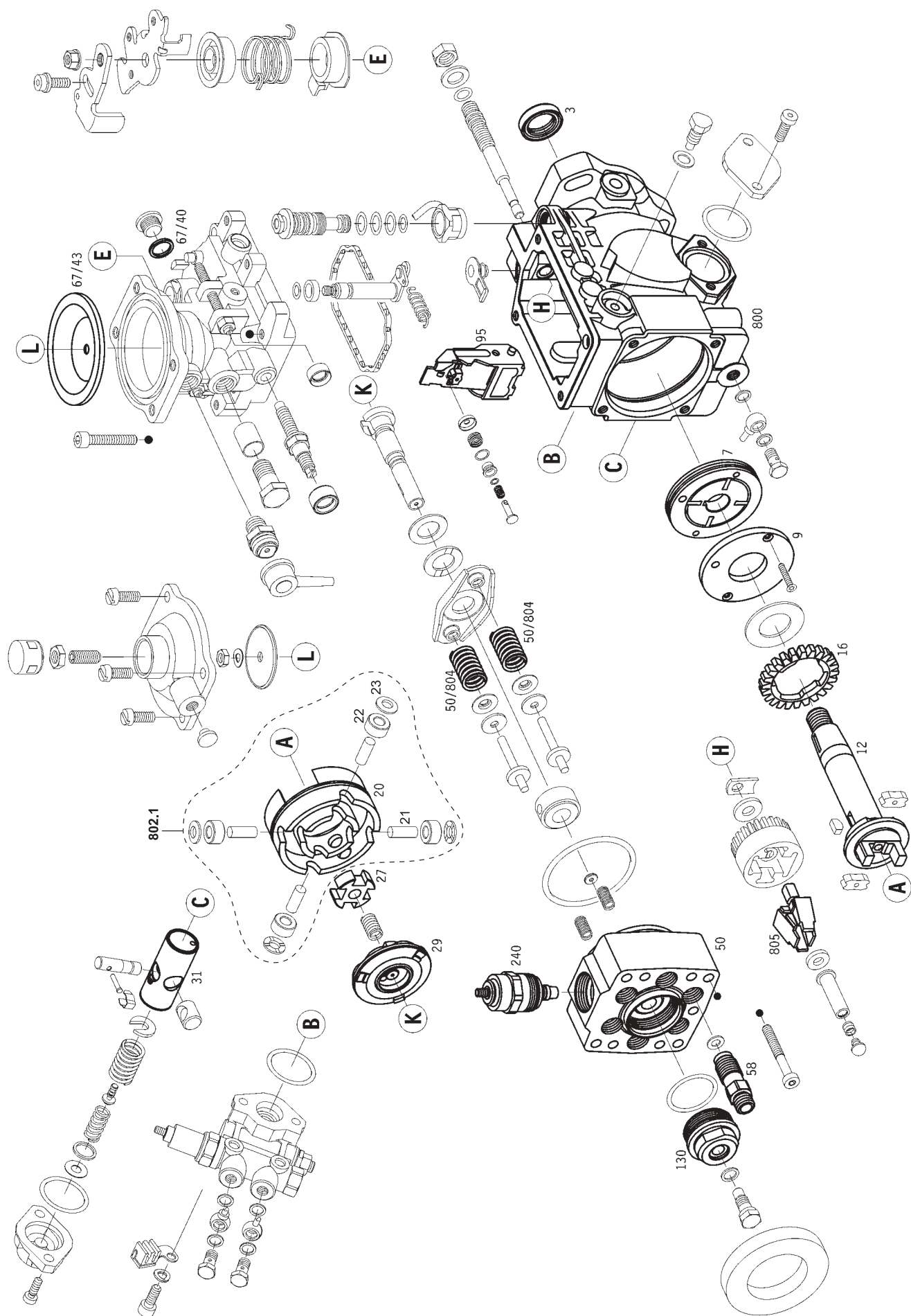
Bomba distribuidora VE: Bomba de inyección rotativa VE:
