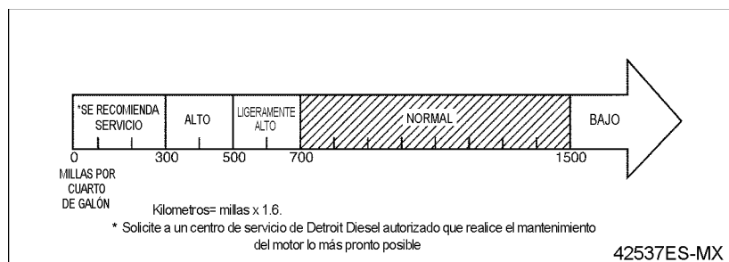
Figure 22 Pautas para el consumo de aceite del motor
