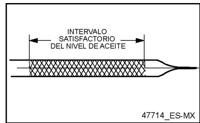
Figure 9 Varilla Medidora de Aceite
