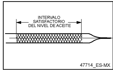
Figure 7 Verifique el Nivel de Aceite Lubricante
