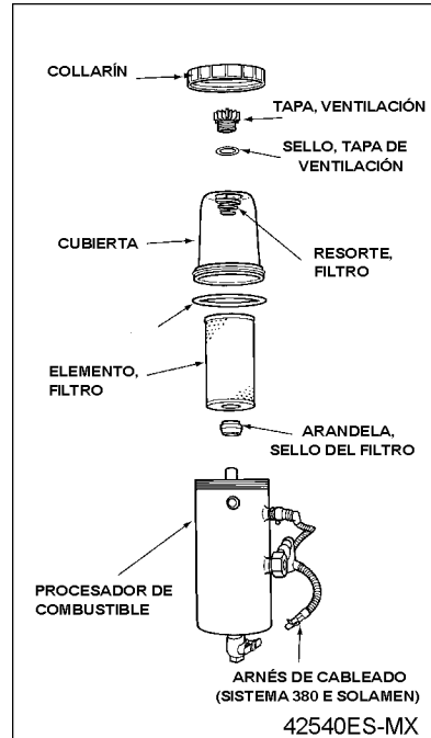
Figure 36 Ensamblaje del procesador de combustible Fuel Pro 382E
