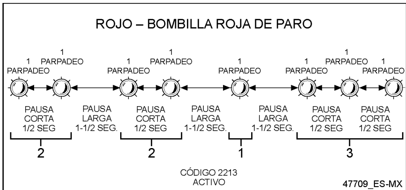
Figure 17 Ejemplo Código de Destello de RSL (Apagar el Motor)
