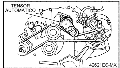
Figure 25 Unidad de tensor de correa automático con alternador 50 DN
