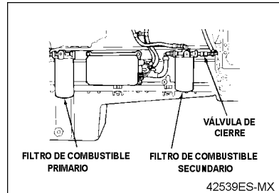
Figure 27 Ubicaciones del Filtro Giratorio de Combustible
